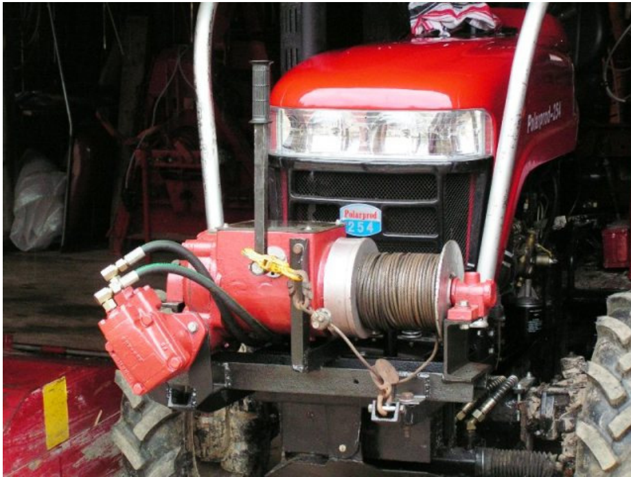
Åtgärd 14. Hydrauldriven frontvinsch. Manövreras från förarsäte alternativt vid vinsch.
